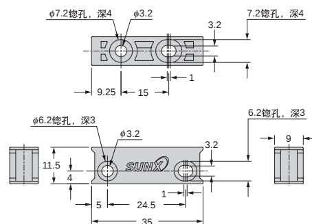
MS-DIN-4 放大器安装支架(另售)
