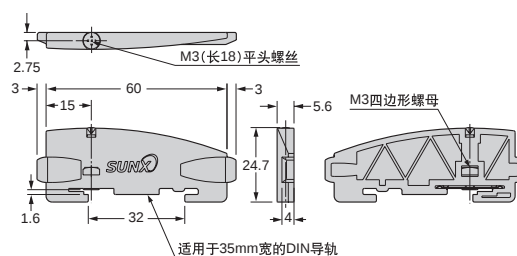
MS-DIN-E 尾盘(另售)
