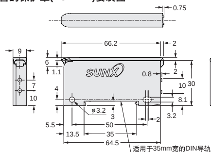
另售的保护罩(FC-FX-1)安装图
