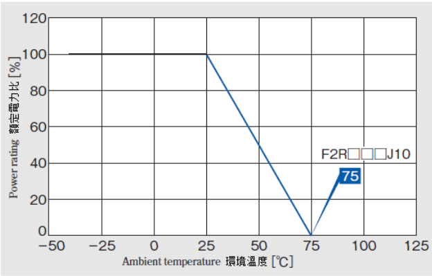
Derating Curve 降低負荷曲線
